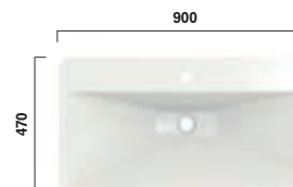
LW172YBT1#XW Möbelwaschtisch SG 900mm, mit Hahnloch, ohne Überlauf Furniture washbasin SG 900mm, with tap hole, without overflow
