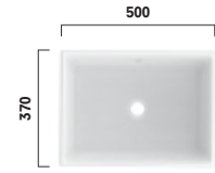
LW1715WH Aufsatzwaschtisch CS, eckig 500mm, ohne Hahnloch, mit Überlauf Vessel CS, square 500mm, without tap hole, with overflow
