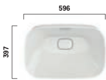
LW3716HY NEOREST Aufsatzwaschtisch 600mm, ohne Hahnloch, mit Überlauf NEOREST vessel 600mm, without tap hole, with overflow
