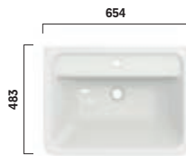
LW136Y Waschtisch CF 650mm, mit Hahnloch, mit Überlauf Washbasin CF 650mm, with tap hole, with overflow
