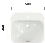
L5615CE Möbelwaschtisch LF 500mm, mit Hahnloch, mit Überlauf Furniture washbasin LF 500mm, with tap hole, with overflow
