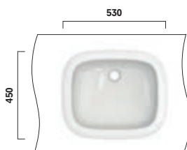
LW763Y Einbauwaschtisch eckig 530mm, ohne Hahnloch, mit Überlauf Self-rim basin square 530mm, without tap hole, with overflow
