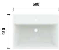
LW1216CKE Waschtisch CS eckig 600mm, mit Hahnloch, mit Überlauf Washbasin CS square 600mm, with tap hole, with overflow
