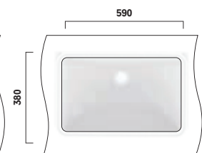
LW1536Y Unterbauwaschtisch WU eckig 600mm, ohne Hahnloch, mit Überlauf Undercounter basin WU square 600mm, without tap hole, with overflow
