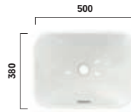
L5715E Aufsatzwaschtisch LF 500mm, ohne Hahnloch, mit Überlauf Vessel LF 500mm, without tap hole, with overflow
