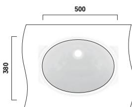
LW1505JUYW/F#W Unterbauwaschtisch WU, rund 500mm, ohne Hahnloch, mit Überlauf Undercounter basin WU round 500mm, without tap hole, with overflow
