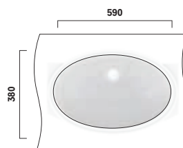
LW1506JUYW/F#W Unterbauwaschtisch WU rund 600mm, ohne Hahnloch, mit Überlauf Undercounter basin WU round 600mm, without tap hole, with overflow
