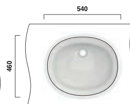
LW764Y Unterbauwaschtisch rund 540mm, ohne Hahnloch, mit Überlauf Undercounter basin round 540mm, without tap hole, with overflow
