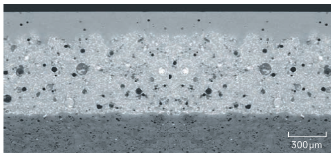
Micrographie WC CEFIONTECT * 1 μm=0,001 mm
