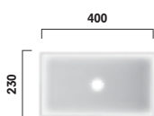
LW1734WH Lave-mains CS, rectangle 400 mm, sans trou, sans trop-plein Lavamani da appoggio CS, rettangolare 400 mm, senza foro per rubinetto e senza troppieno
