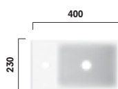
LW1634WH Lave-mains CS, rectangle 400 mm, percé un trou, sans trop-plein Lavamani da appoggio CS, rettangolare 400 mm, con foro per rubinetto e senza troppieno
