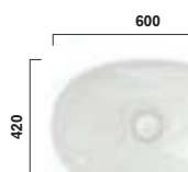
L4706E#XW Vasque TL rond 600 mm sans trou, sans trop-plein, avec écoulement libre Lavabo TL rotondo 600mm, senza foro per rubinetto, senza troppieno, con piletta
