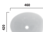
L4704E Lavabo TA, asymétrique 460mm, sans trou, avec trop-plein Lavabo TA asimmetrico 460mm, senza foro per rubinetto, con troppieno
