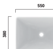
L1735E Lavabo WU rectangle 600mm, sans trou, avec trop-plein Lavabo WU rettangolare 600mm, senza foro per rubinetto, con troppieno
